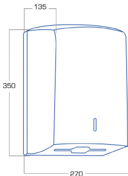
Dimensiones.
